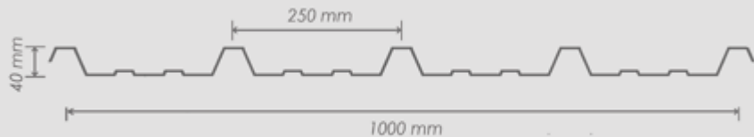
Lichtdoorlatende POLYCARBONAAT platen TC 40-250-4
