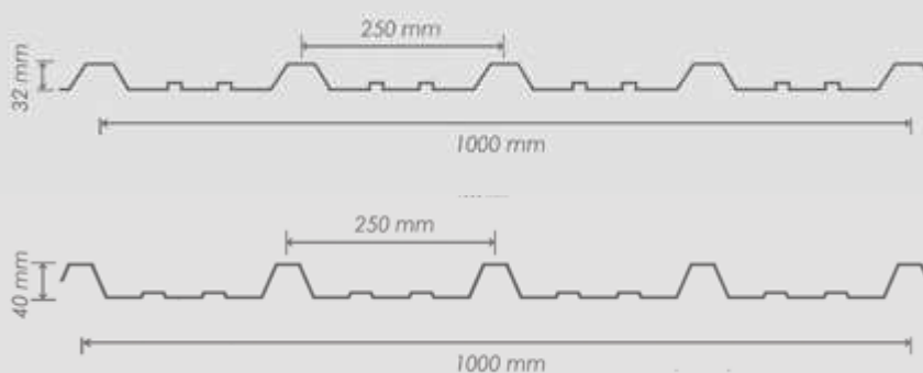
LICHTDOORLATENDE PLATEN POLYESTER TC 32-250-4 en TC 40-250-4
